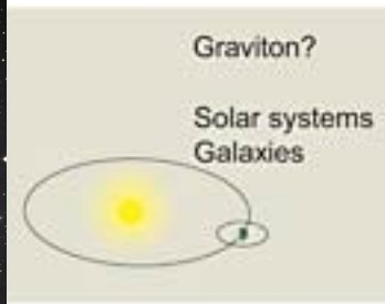
Force gravitationnelle
