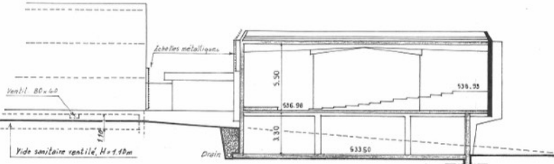
Coupe A.A.
