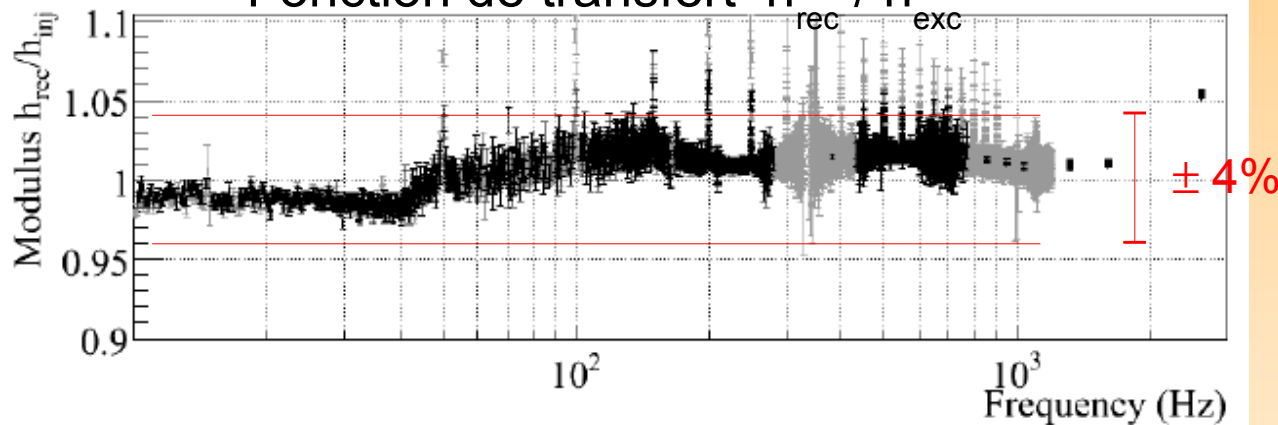
Fonction de transfert h_{\text{rec}} / h_{\text{exc}}
