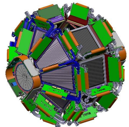
Enceinte GRIT : Dext 450 mm Dint 444 mm
