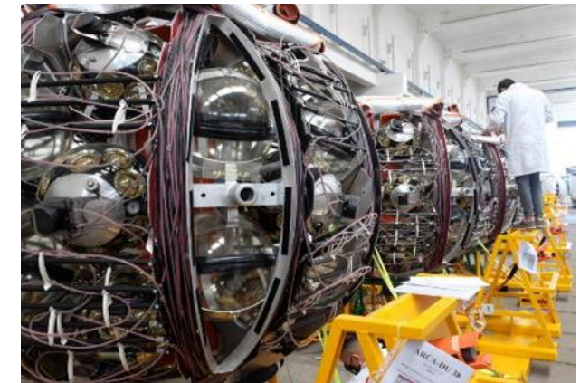
Intégration des lanceurs
