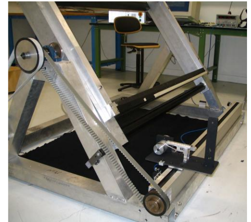
Outillage de tissage de fils sur les cadres de transfert
