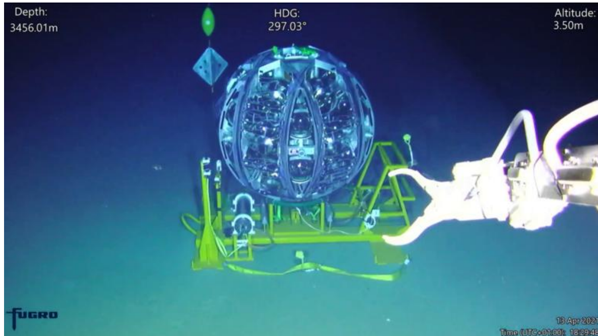
Connexion avec l'aide d'un ROV (véhicule sous-marin téléopéré)
