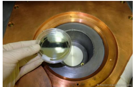
Partie active du détecteur Ge
