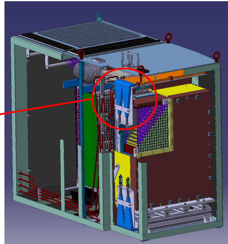
Calorimètre NPS
