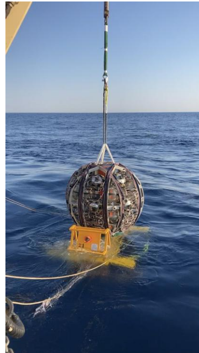
Mise à l'eau des lanceurs
