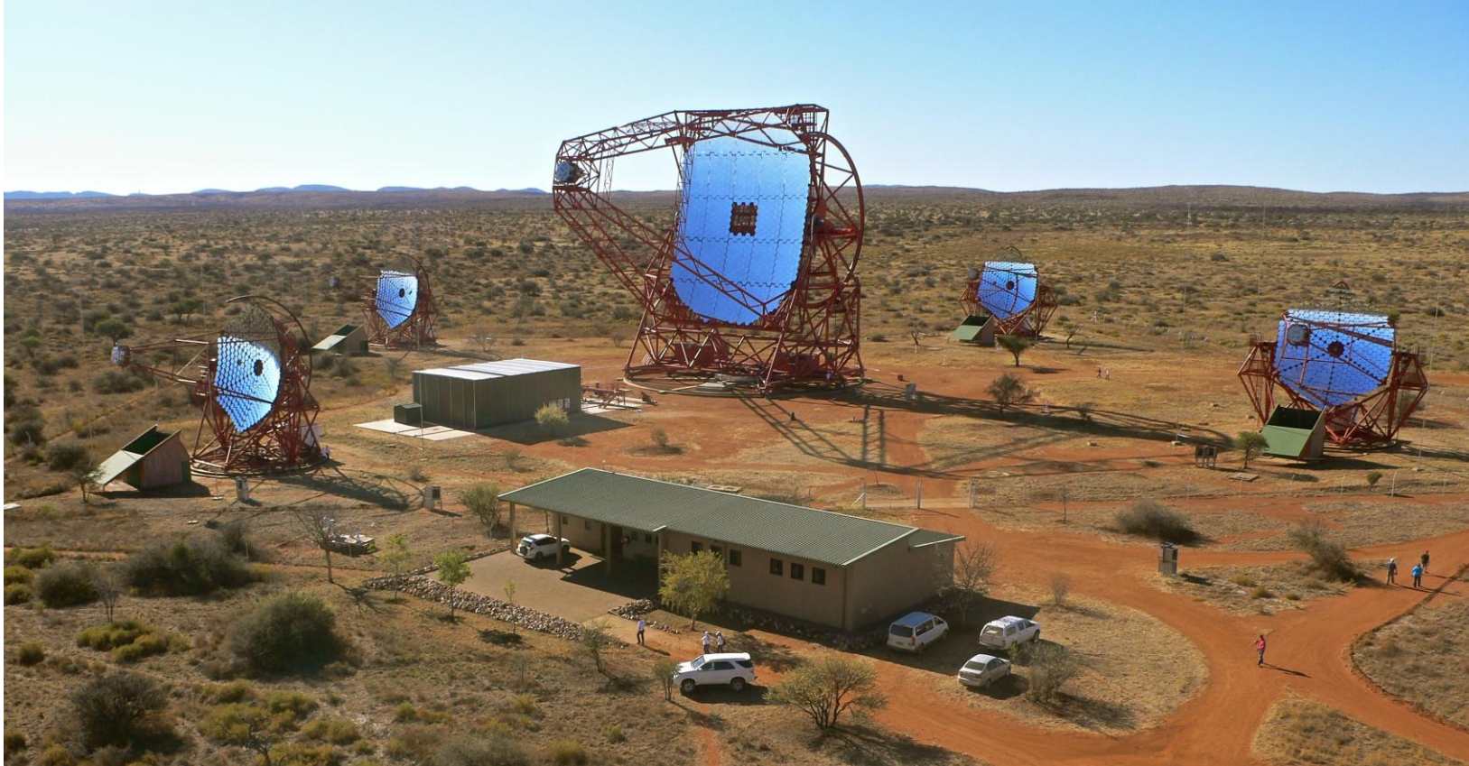
Expérience HESS
