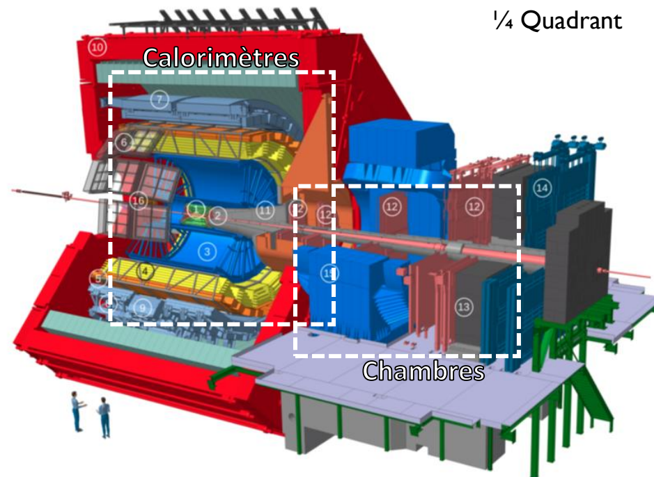
Expérience ALICE
