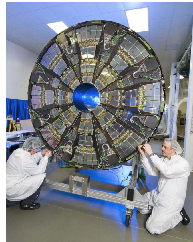
Un disque du tracker de CMS
