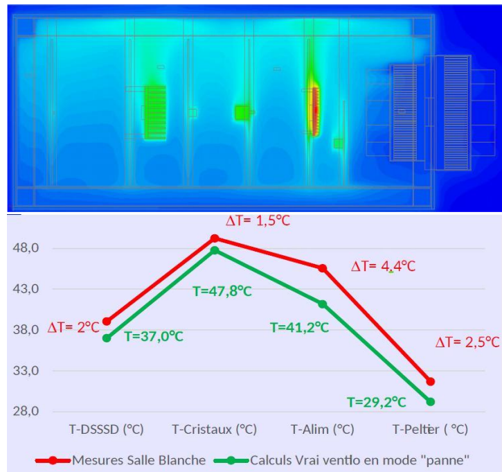
Sans ventilateur et sans Peltier
