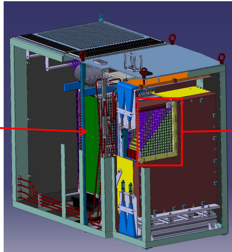
Calorimètre NPS
