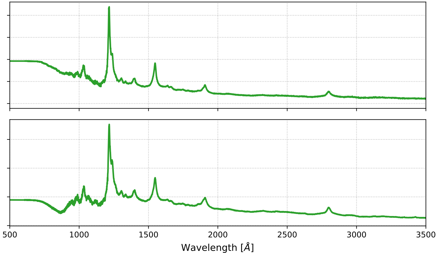
Quasi Stellar Object (Quasar)
