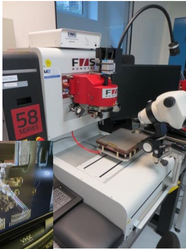
Machine à bonder (micro-connexions) Bonding machine (micro-interconnects)
