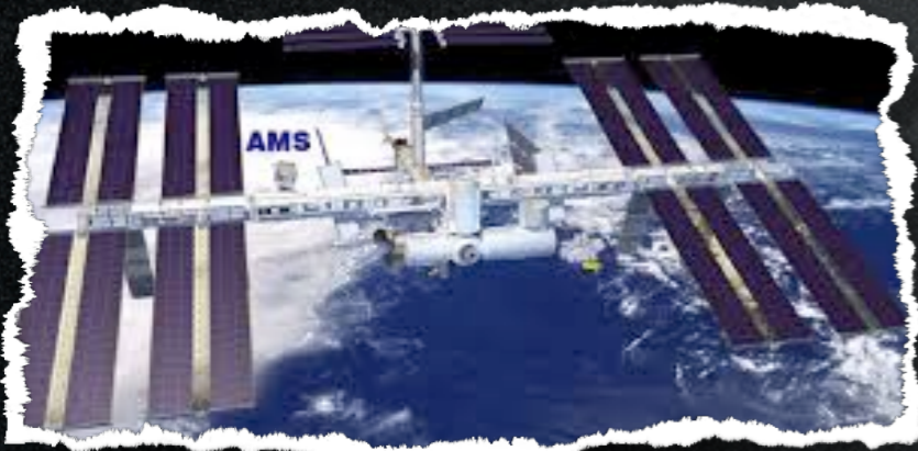
Physique spatiale
