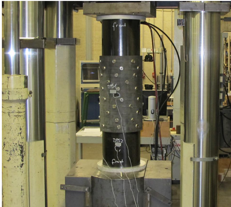
Test de compression (250 tonnes)
