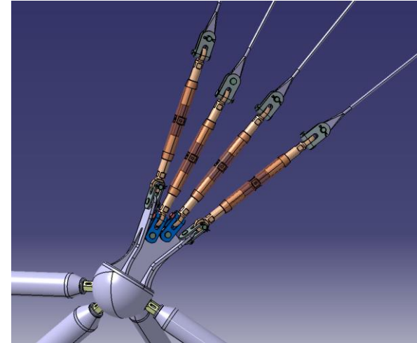
Ancrage et mise en tension des haubans du télescope
