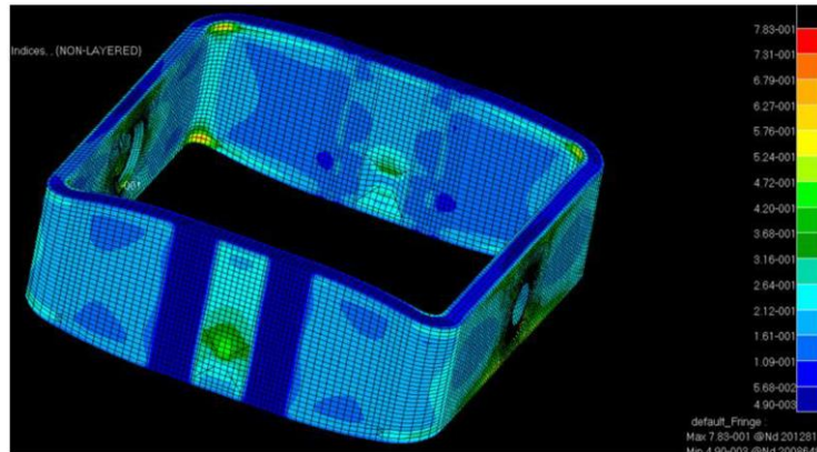
Cadre de liaison de l'arche du télescope
