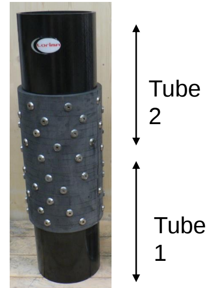
Manchon de jonction de 2 tubes
