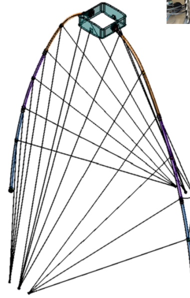
Arche haubanée
