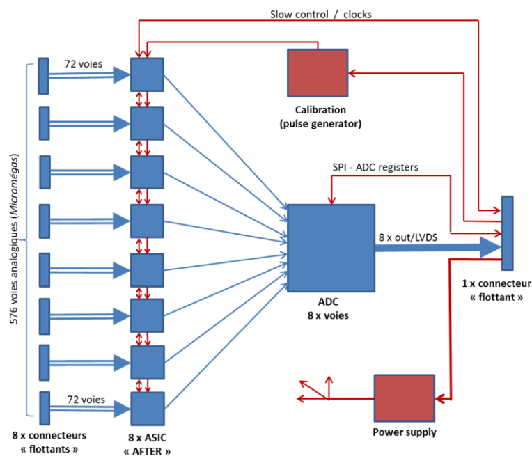
Figure 3-1: Synoptique de fonctionnement de la carte électronique FEC
