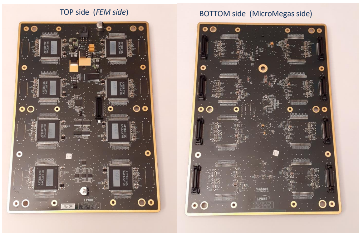
Figure 3-2: Carte électronique FEC
