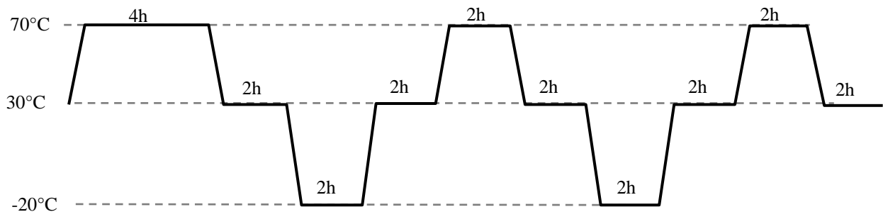
Figure 6-1 : Profil en température du déverminage
