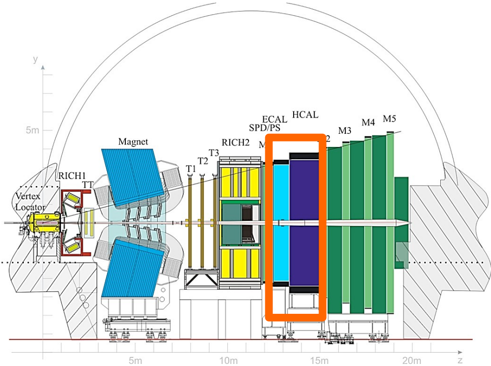
Les calorimètres
