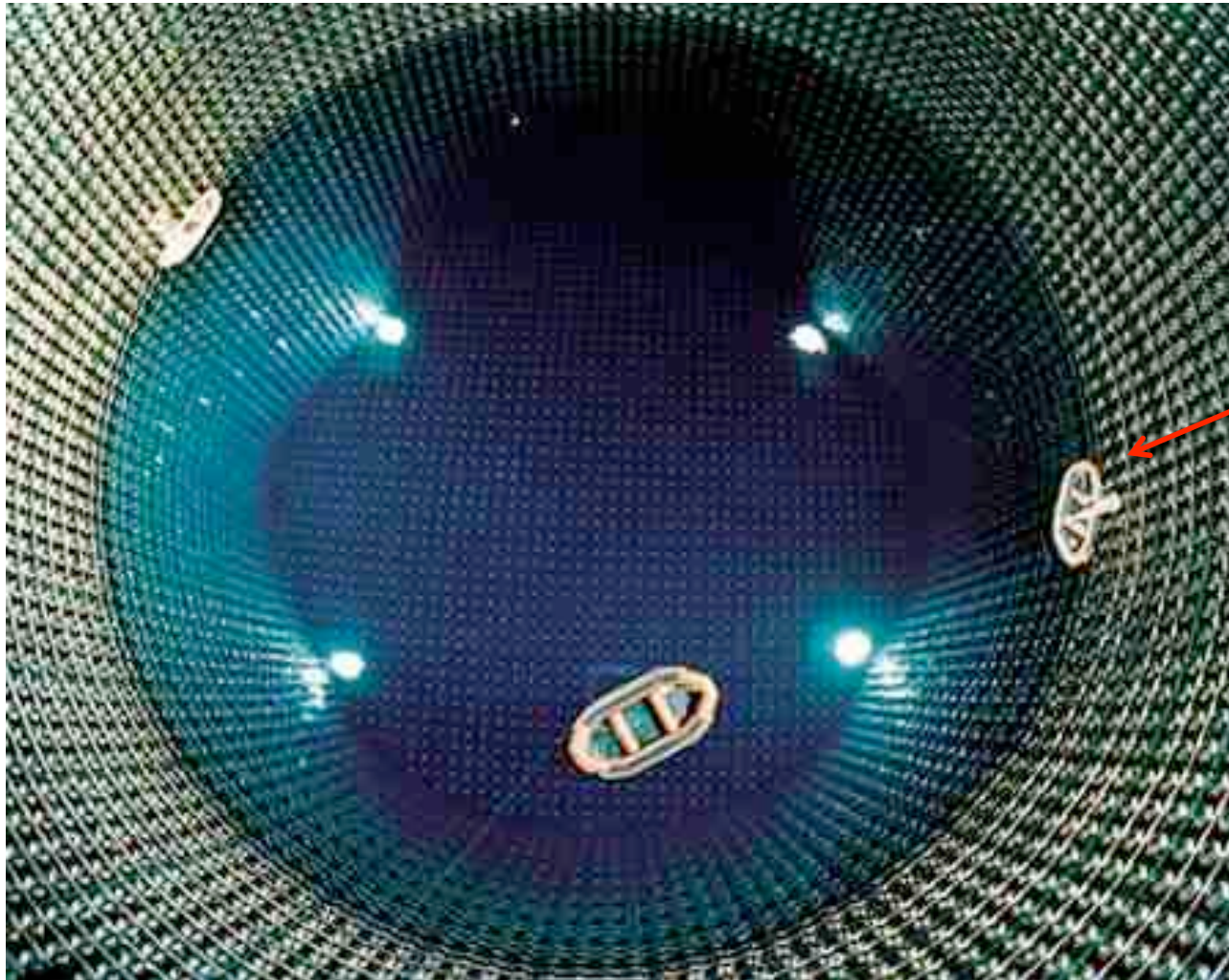
Physiciens sur bateau gonflable inspectant les capteurs
