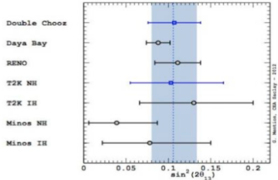
Comparaison des derniers résultats de mesure de l'angle de mélange \theta_{13} par les expériences auprès de réacteurs (Daya Bay, Double Chooz, RENO) et auprès d'accélérateurs (Minos, T2K). La bande bleue est la combinaison des résultats des expériences de l'Irfu, Double Chooz et T2K.
